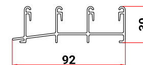
Rälsprofil 4-spår
