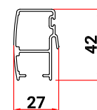
Vertikal luckprofil
