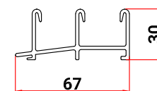
Rälsprofil 3-spår
