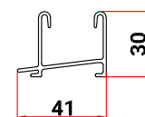
Rälsprofil 2-spår
